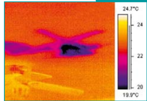
Innenaufnahme einer durchfeuchteten Decke
