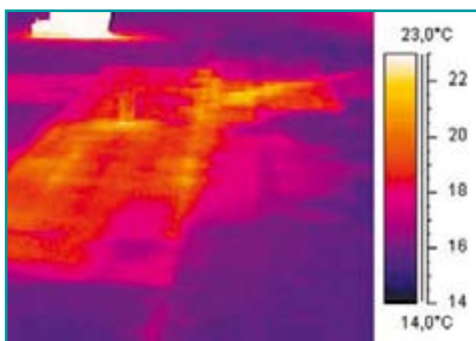
Flachdach mit Regenwassereinschluss
