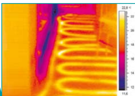
Heizspiralen einer Fußbodenheizung
