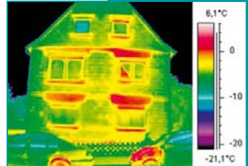
Wärmeverlust durch nicht gedämmte Rolladenkästen
